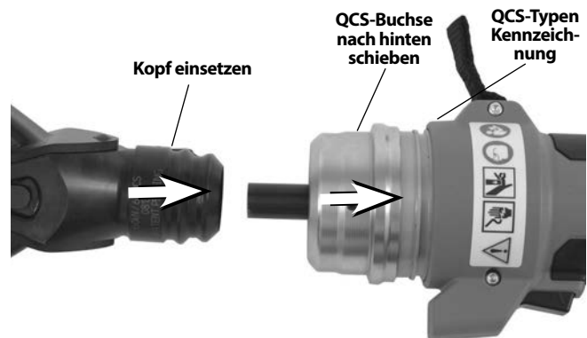
Abbildung 10 – Einsetzen des Wechselkopfes in die QCS-Kupplung
